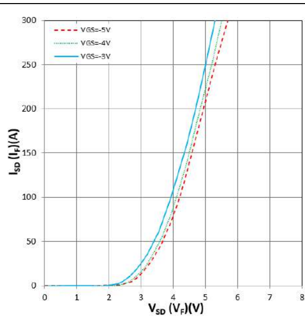
Figure 8. I_{SD} vs V_{SD} ( V_F ) T_j = 150^\circ\text{C} , V_{GS} parameter
